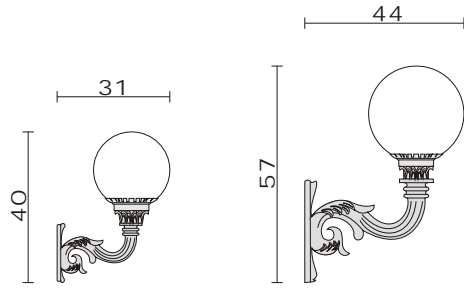
Kugel Ø 20 max. 60 Watt 8400
