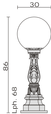
Kugel Ø 30 (Halter Art.Nr. 809) max. 75 Watt
